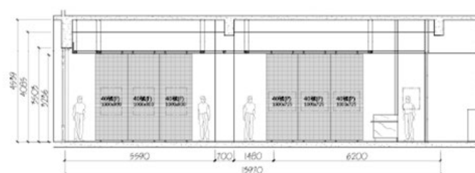
圖 21.23-3 藝文中心立面圖
